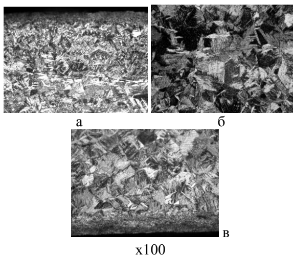
Рис. 3. Мікроструктура сплаву Grade 9 після пресування й охолодження на повітрі (а – зовнішня поверхня, б – середина, в – внутрішня поверхня)
