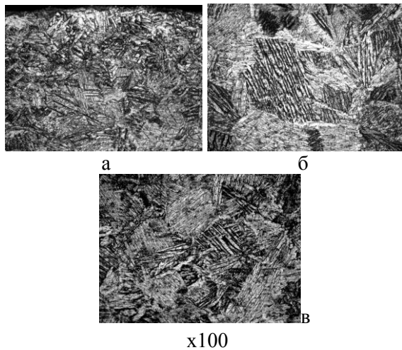
Рис. 2. Мікроструктура труб зі сплаву ПТ-1М після пресування й охолодження у воді (а – зовнішня поверхня, б – середина, в – внутрішня поверхня)
