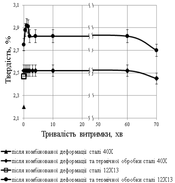
Рис. 1. Залежність твердості від тривалості витримки передрекристалізаційної термічної обробки деформованих сталей 40X та 12X13
