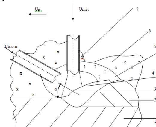
Рис.1. Схема наплавки под флюсом порошковой проволокой с подачей обесточенной присадки: U_{п.} – скорость наплавки, м/ч; U_{п.э.} – скорость подачи электрода, м/ч; U_{п.о.п.} – скорость подачи обесточенной присадки, м/ч; \alpha – угол подачи обесточенной присадки; 1 – основной металл; 2 – наплавленный металл; 3 – дуговой промежуток; 4 – жидкий металл; 5 – жидкий шлак; 6 – шлак; 7 – флюс
