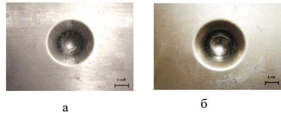
Рис. 4. Зразки після випробувань на видавлювання: а – вихідний до ІБ; б – після ІБ з двох сторін
