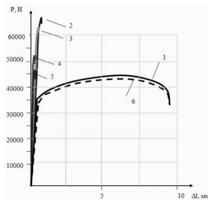
Рис. 1. Криві розтягання зразків сталі 20: 1 – після Г+ Н.В.; 2 – цементация на глибину 0,5 мм; 3 – 1,0 мм; 4 – 1,5 мм; 5 – 2,0 мм; 6 – після зняття шару цементации
