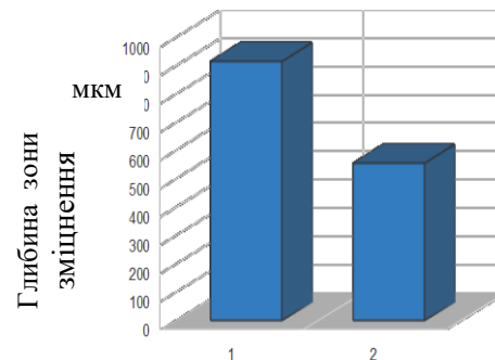
Рис. 6. Результати вимірювання глибини зони зміцнення сталі 9XC після комплексного обробки (азотування, гартування і відпуску) за режимами 2 і 3 (1 – відпуск 150 °С), (2 – відпуск 250 °С)
