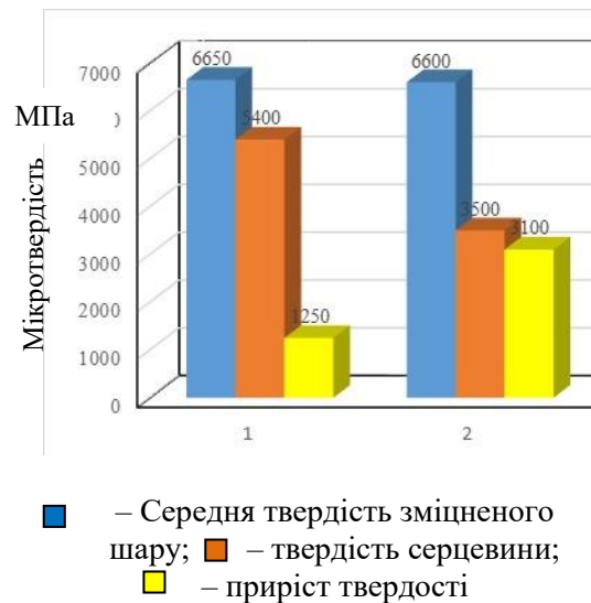
Рис. 5. Результати вимірювання мікротвердості сталі 9XC після комплексного обробки (азотування, гартування і відпуску) за режимами 2 і 3 (1 – відпуск 150 °С), (2 – відпуск 250 °С).
