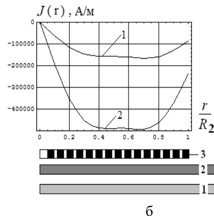
Рис. 3. Распределение индуцированных токов в стальной заготовке и экране при частоте f=5000 Гц, \varphi_{m1} = 1,099 рад и \varphi_{m2} = 0,942 рад
