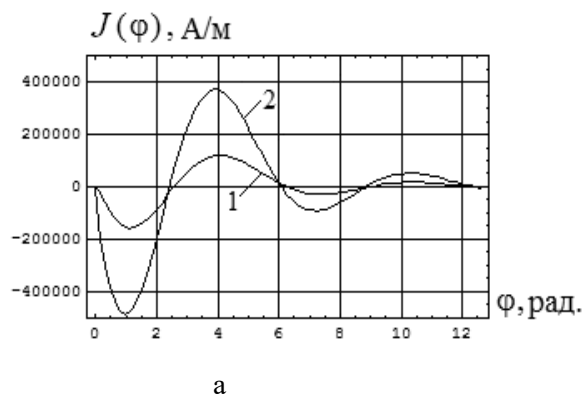
Рис. 3. Распределение индуцированных токов в стальной заготовке и экране при частоте f=5000 Гц, \varphi_{m1} = 1,099 рад и \varphi_{m2} = 0,942 рад
