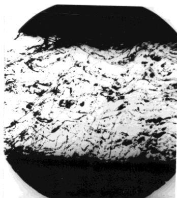
Рис. 1. Микроструктура сталь-молибденового покрытия ×115
