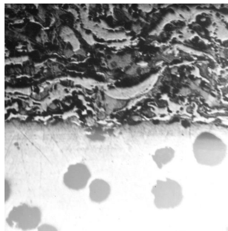
Рис. 2. Микроструктура сталь-молибденового покрытия в травленном состоянии, x115
