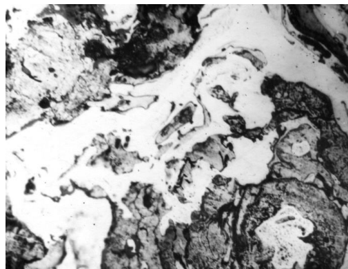
Рис. 3. Микроструктура поверхностного слоя стале-молибденового покрытия, ×400
